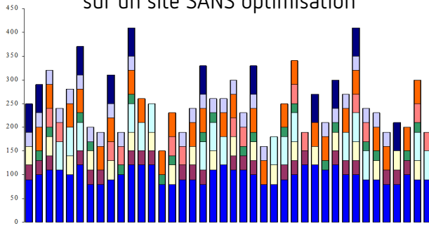
Puissance intégrée par période sur un site SANS optimisation
